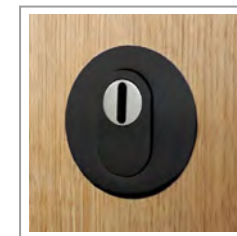
SZAP PLANO - Varnostna rozeta s pokrivalom za cilinder, nerjavno jeklo črna mat (debelina 1mm)
