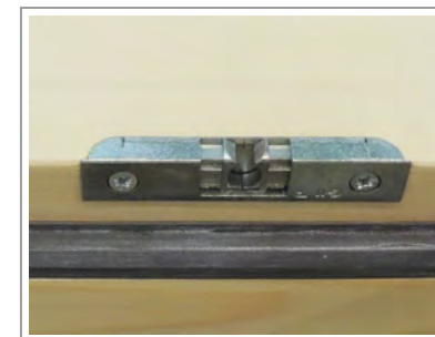
ZASKOČNIK dodatni zaustavljalac vrat pri izvedbah z dan/noč funkcijo (EP, AV3, EAV3)
