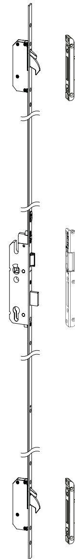
AV3 Avtomatik z dan / noč stikalom 3 - točkovno zaklepanje 2 kavlja, Začasno lahko s stikalom blokiramo delovanje magnetnega sprožilca, ki omogoča avtomatsko pomikanje kavljev
