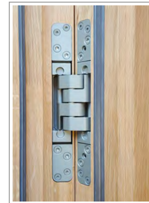
SKRITA NASADILA (standardno samo pri poravnani izvedbi vrat) 3D nastavljiva, nosilnost 180 kg, srebrna barve
